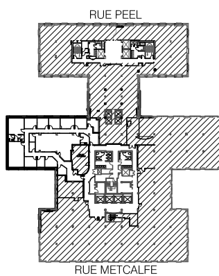
PLAN CLÉ
